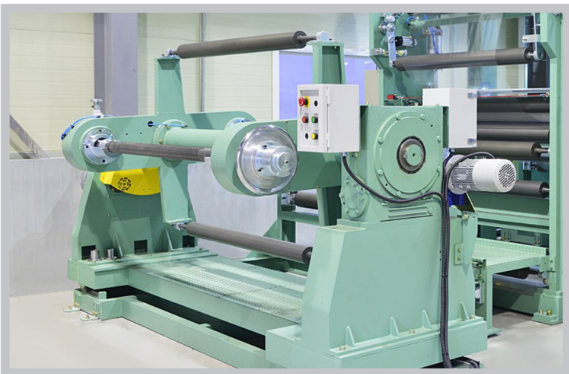
①⑦ UN WINDER
